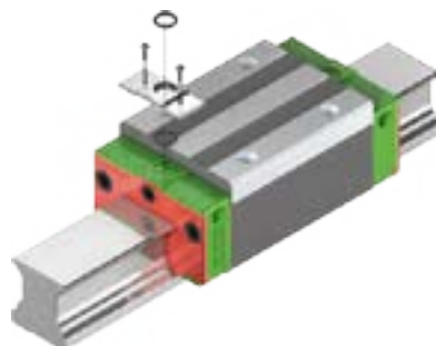
Fig. 5.4 Raccordo di lubrificazione in alto (HG, CG, RG)
