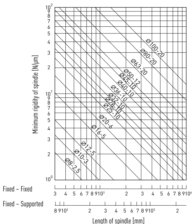
Fig. 3.26 Grafico della rigidezza alberi
