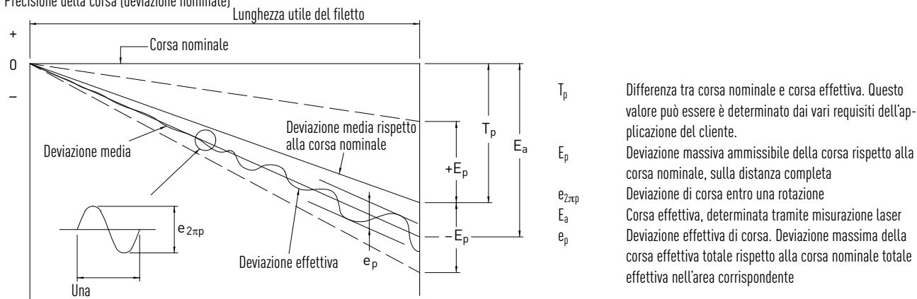
Fig. 3.12 Misurazione HIWIN dell'errore del passo per le viti a ricircolo di sfere di precisione
