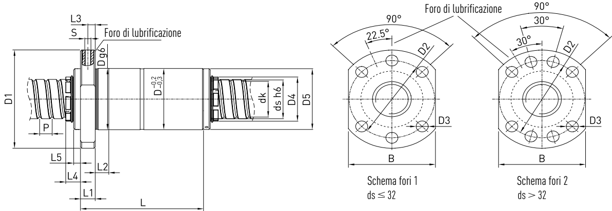
Fig. 5.3 Chiocciole flangiate doppie DDB con tenute NW e SP
