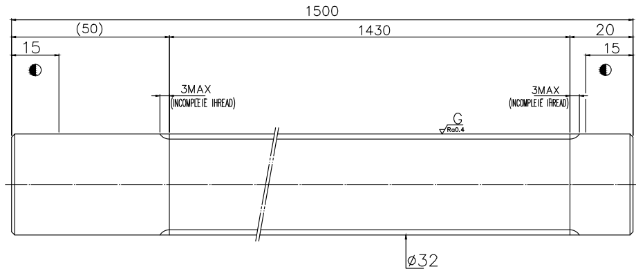
Esempio di albero a stock R32-10-1430-1500-0,018
