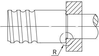
Fig. 3.7 Scarico R per l'alloggiamento del cuscinetto
