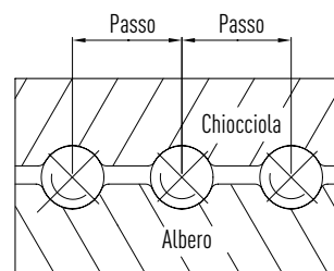
Fig. 3.18 Precarico con sfere maggiorate
