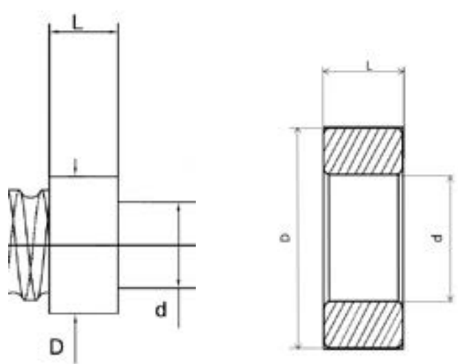
Anello calettato sull'albero
