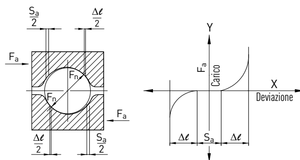
Fig. 3.17 Profilo ad arco gotico e precarico
