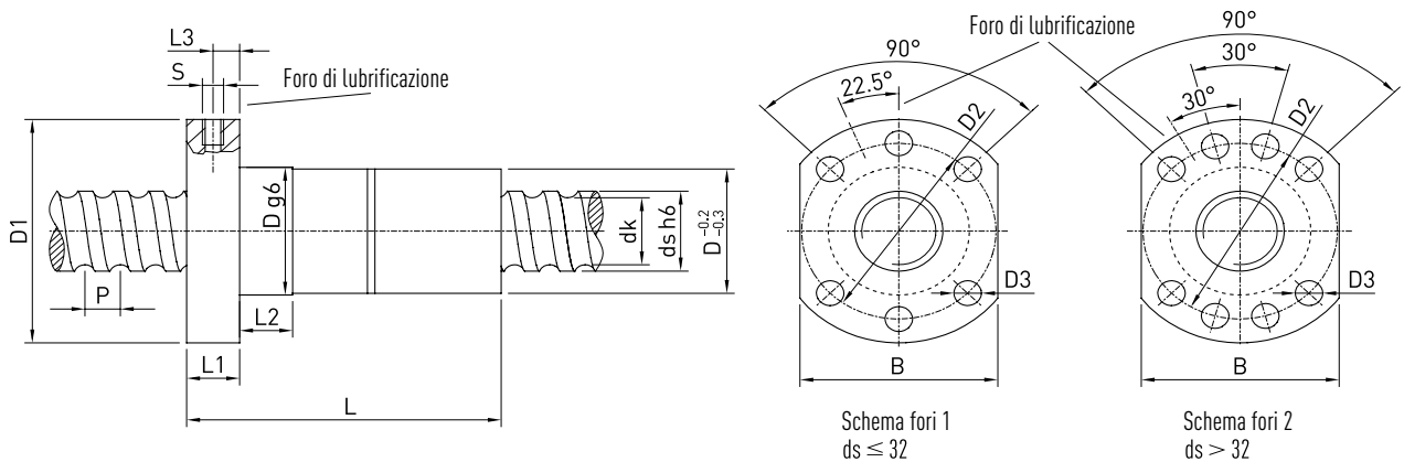
Fig. 5.3 Chiocciole flangiate doppie DDB con tenute NW e SP
