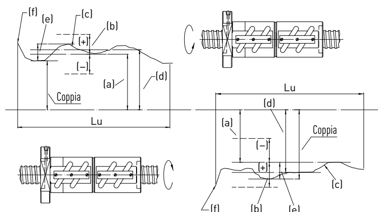
Fig. 3.21 Nomenclatura per la misurazione delle coppie resistenti
