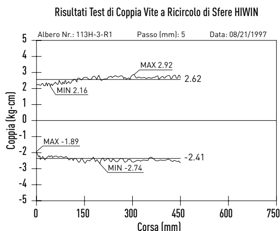
Fig. 2.4 Controllo HIWIN del precarico
